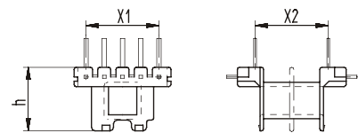
Рис. 2 Горизонтальный каркас
