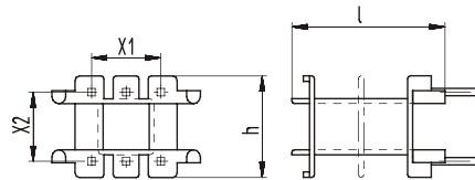
Рис. 1 Вертикальный каркас
