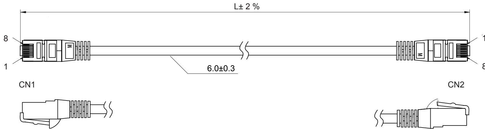
PIN-Belegung/PIN out
