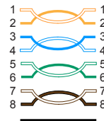
PIN-Belegung/PIN out
