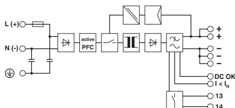
Блок-схема
