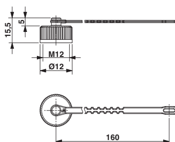
Чертеж
