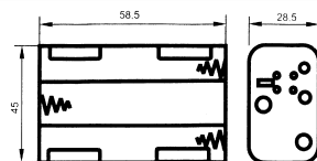
ВН-623 на 4 элемента "AAA"
