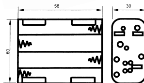
ВН-625 на 4 элемента "AAA"
