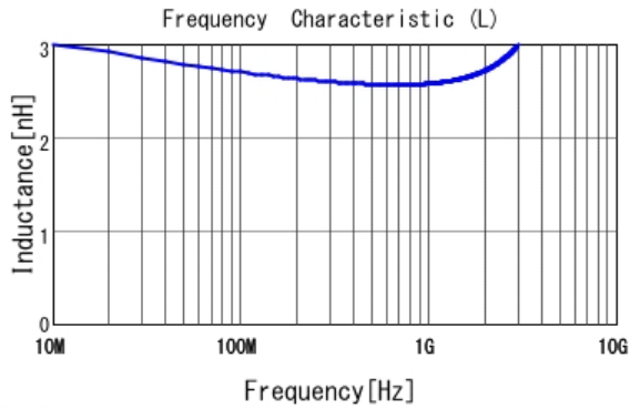
■ LQG15HS2N7S02 L
