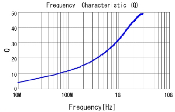
■ LQG15HS2N7S02 Q
