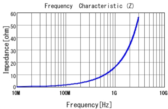
■ LQG15HS2N7S02 |Z|
