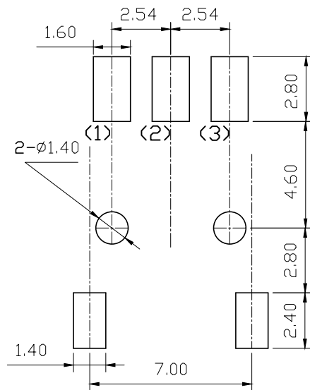
P.C.B. DIMENSION
