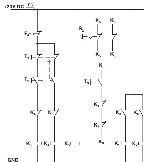
Станд. схема соединения Цепь управления реверс. контактора кат. 3
