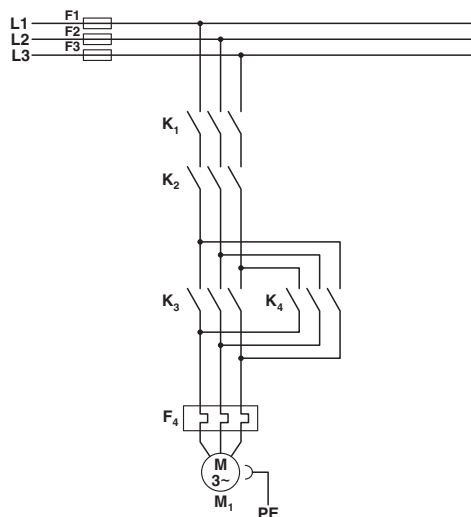
Стандартная схема соединения Цепь питания реверсивного контактора кат. 3
