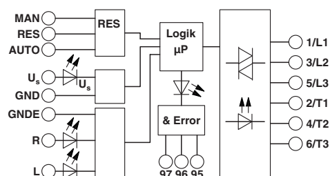
Блок-схема
