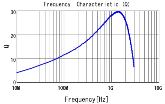
■ LQG15HS12NJ02 Q
