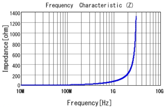
■ LQG15HS12NJ02 |Z|
