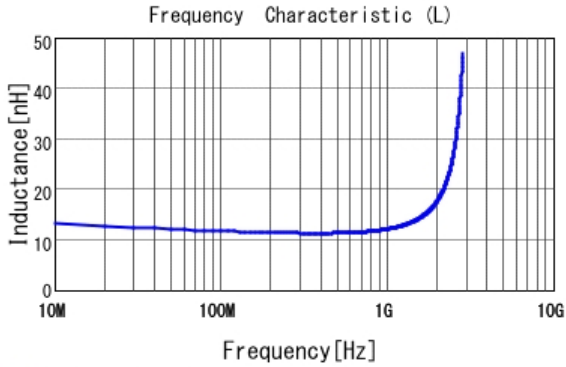
■ LQG15HS12NJ02 L
